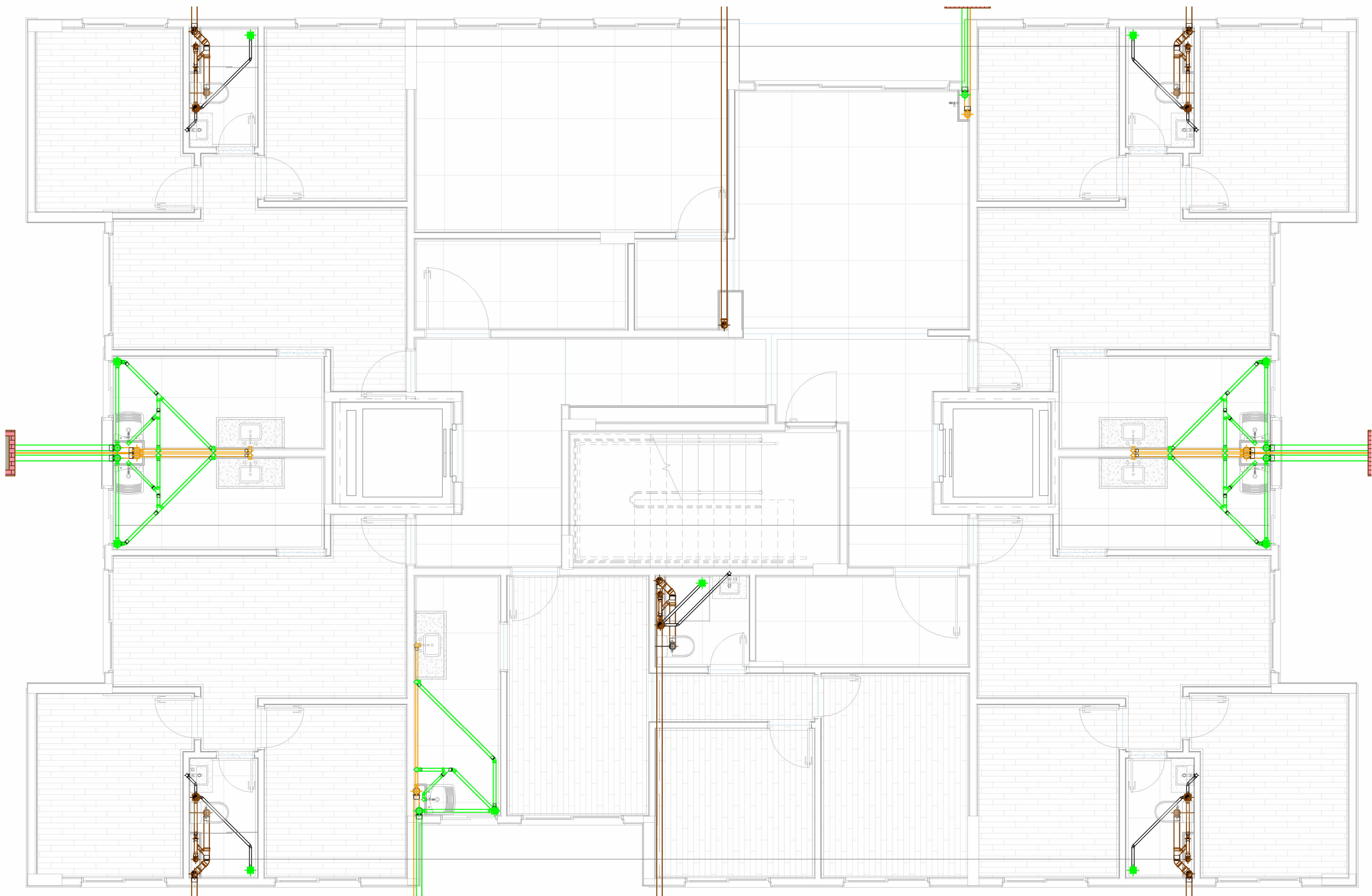
Pavimento Tipo 1 1 : 50
