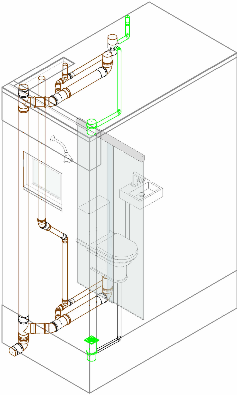
ISO - Banheiro 1
