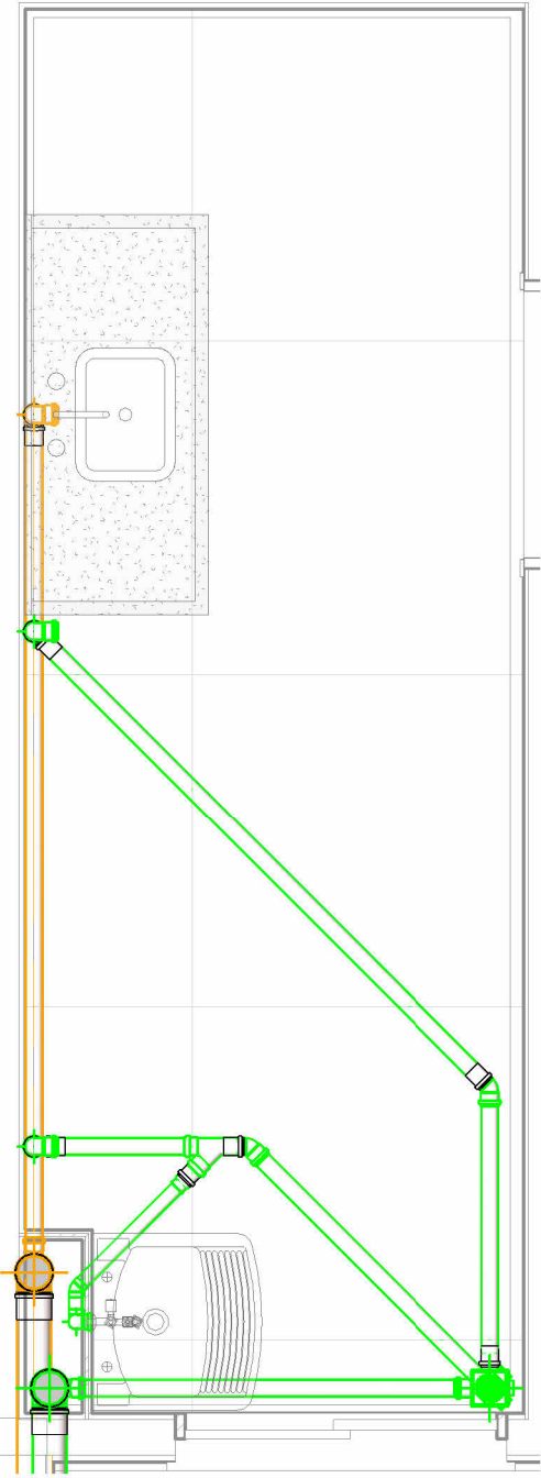
Cozinha 2 1 : 25
