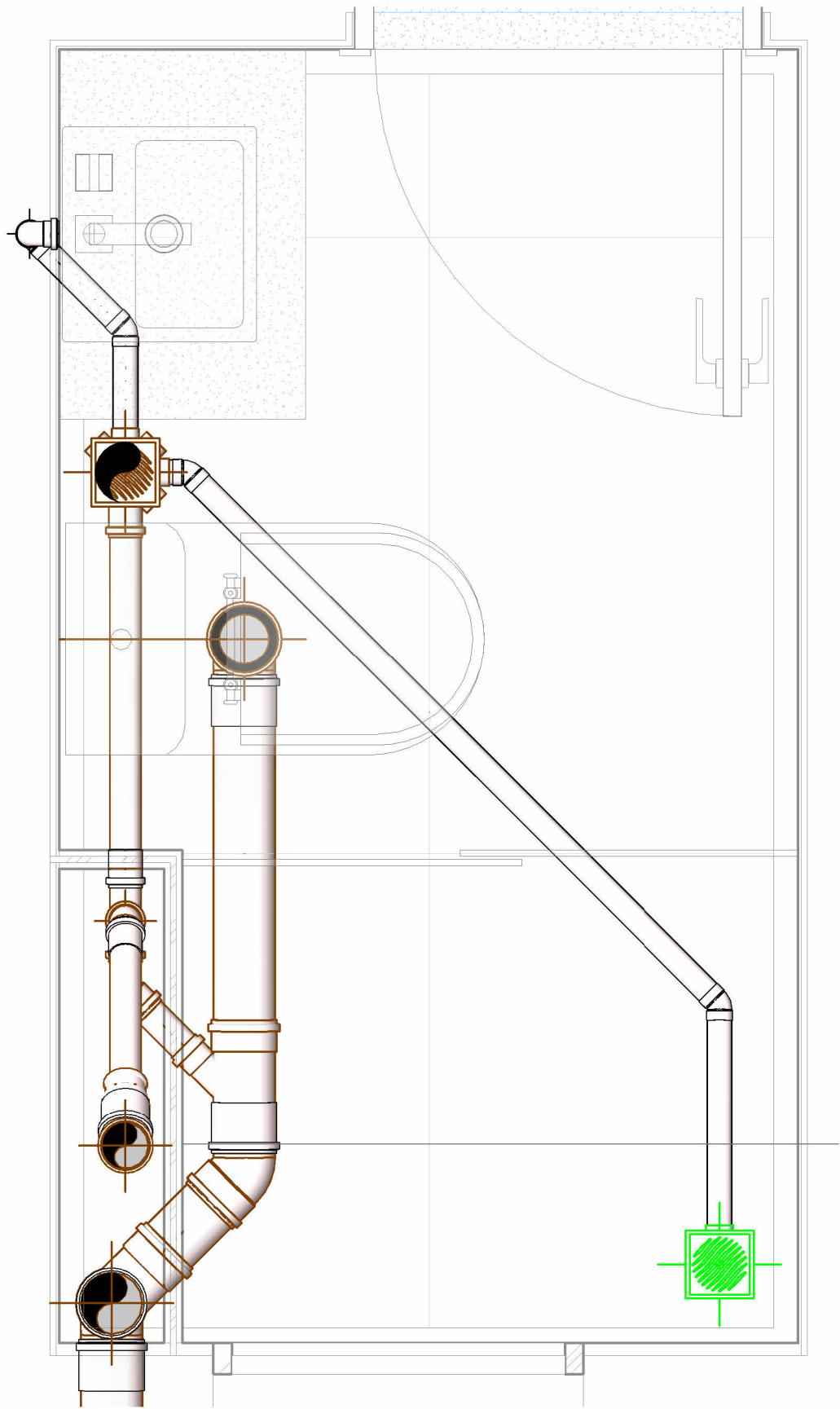
Banheiro 1
