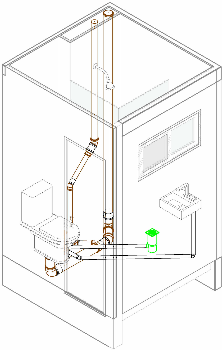
ISO - Banheiro 2
