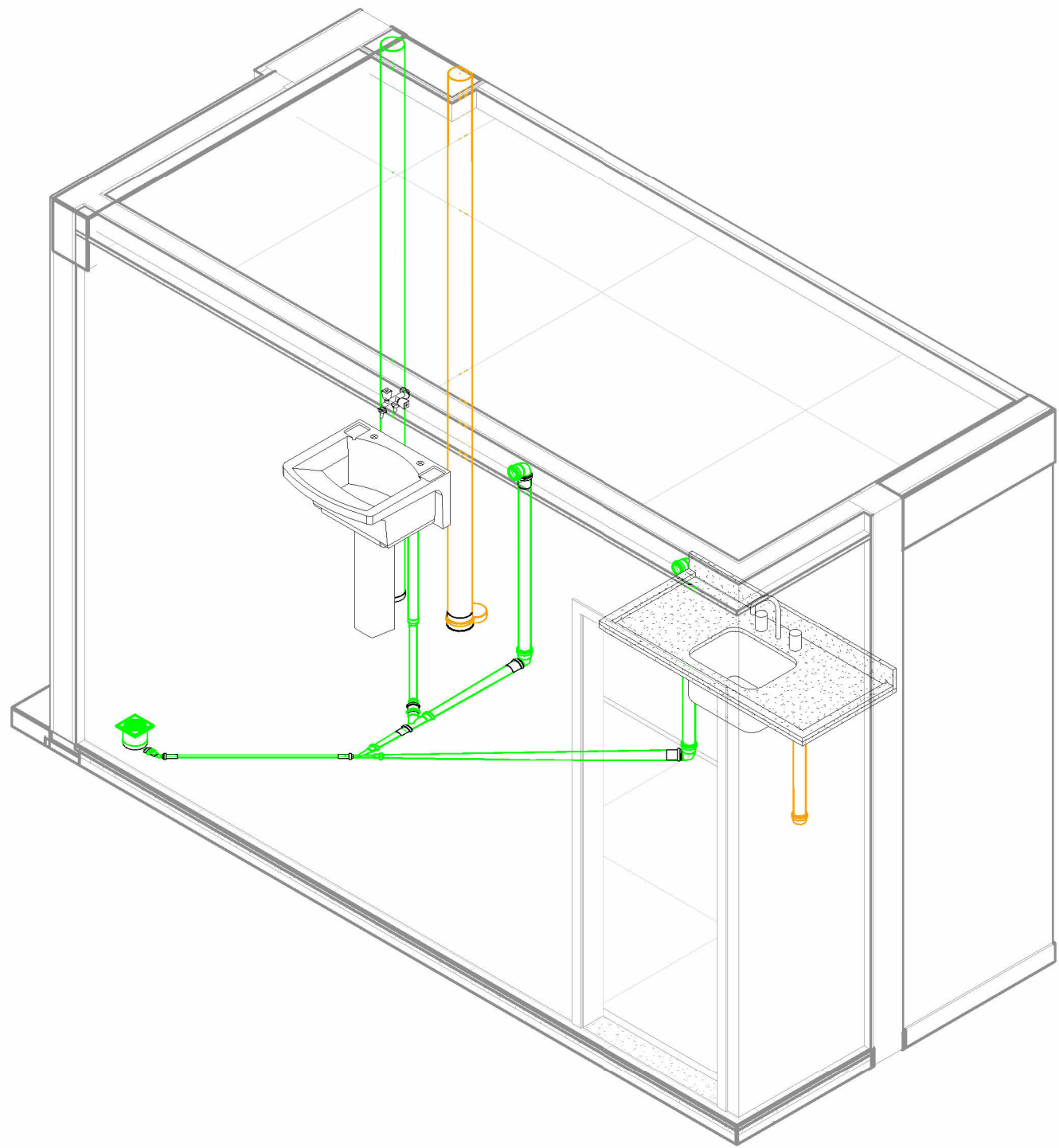
ISO - Cozinha 1
