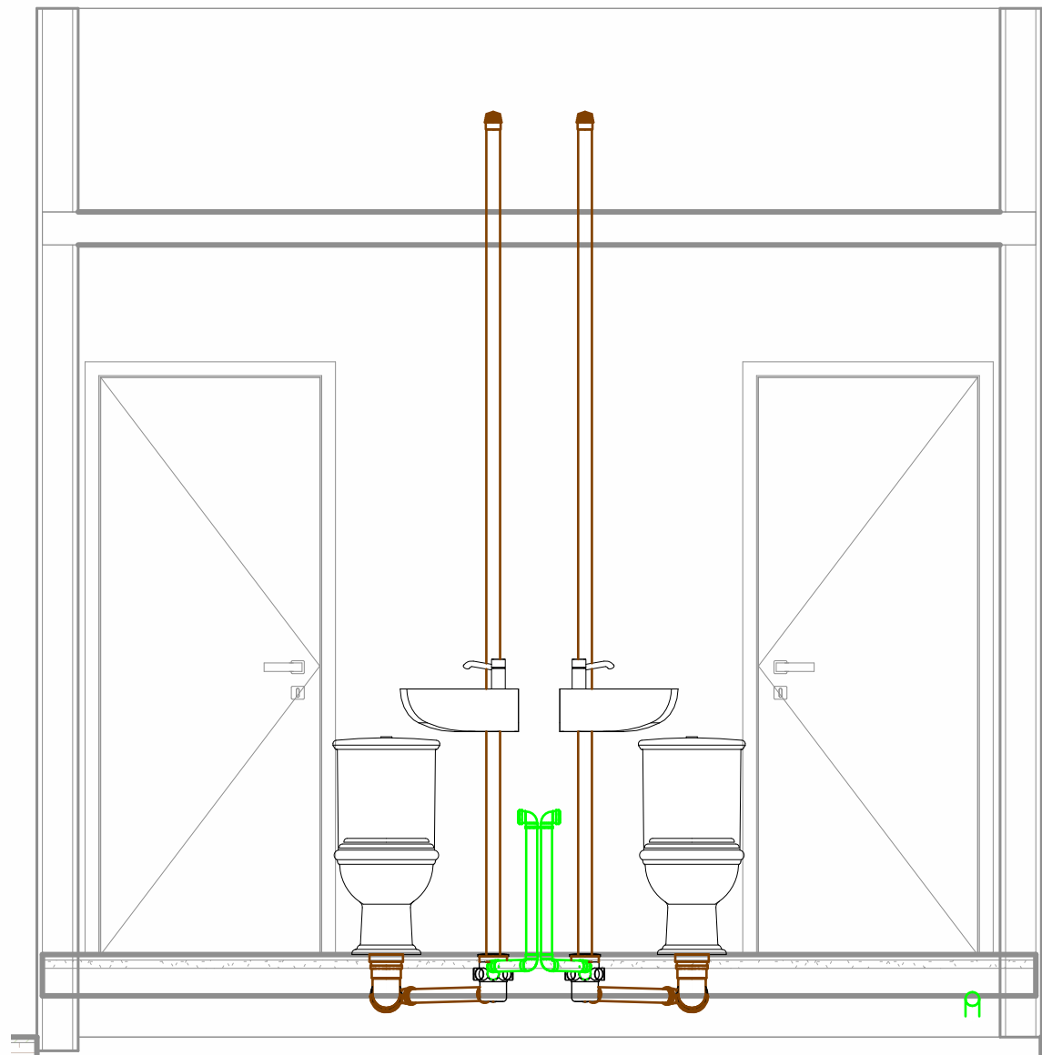
Banheiros
