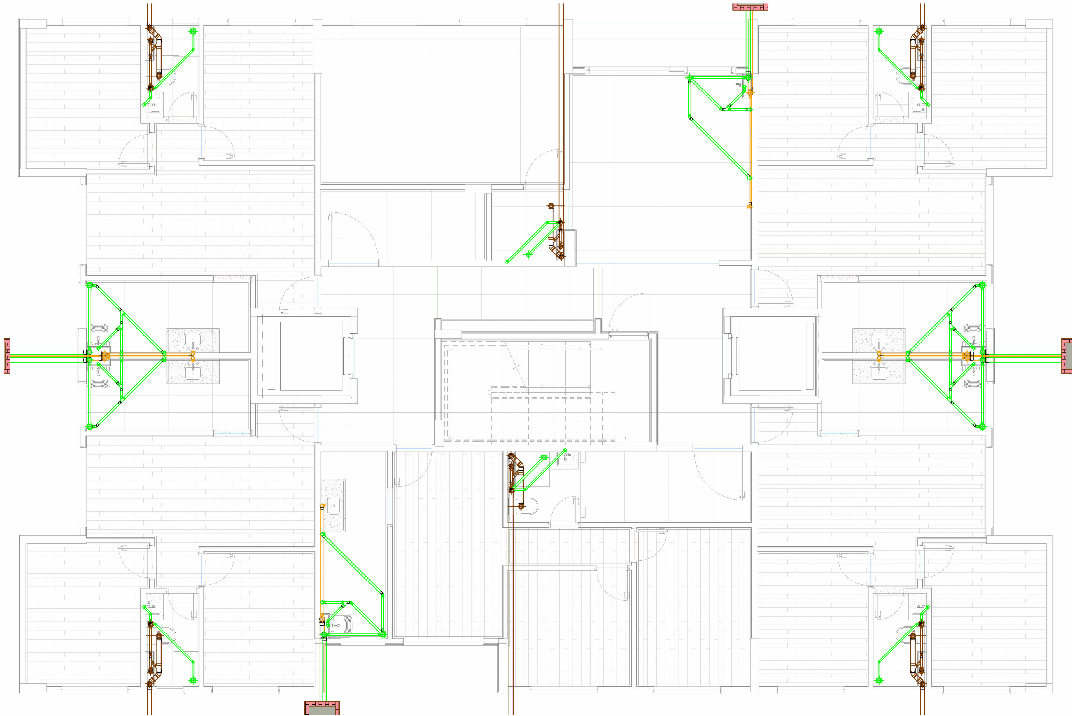
Pavimento Tipo 2
