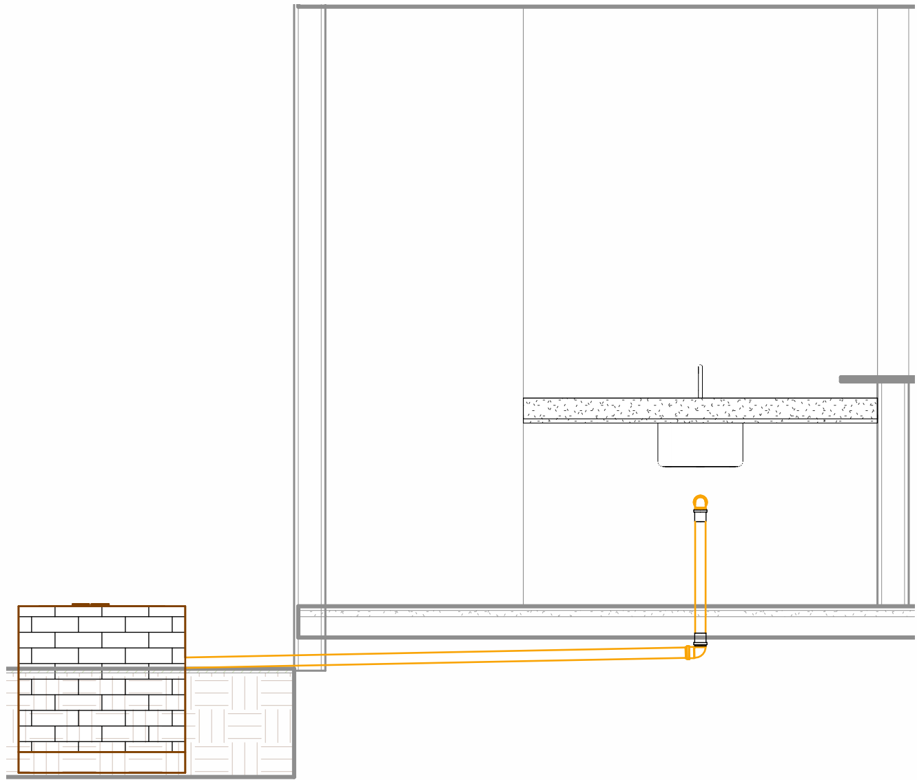
Cozinha
