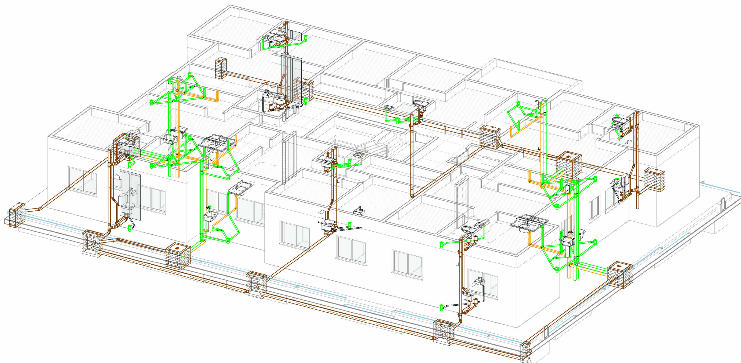
ISO - Pavimento Tipo 1
